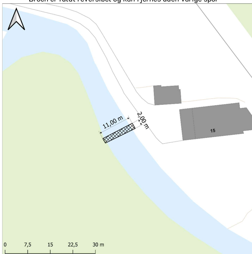
Figur 2: Broens placering og vejledende dimensioner.
