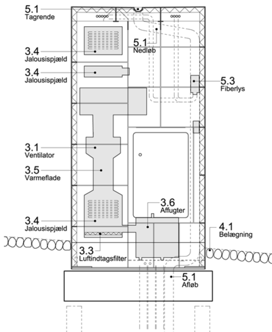
PRINCIPSNIT I LILLE AFSKÆRMNING
