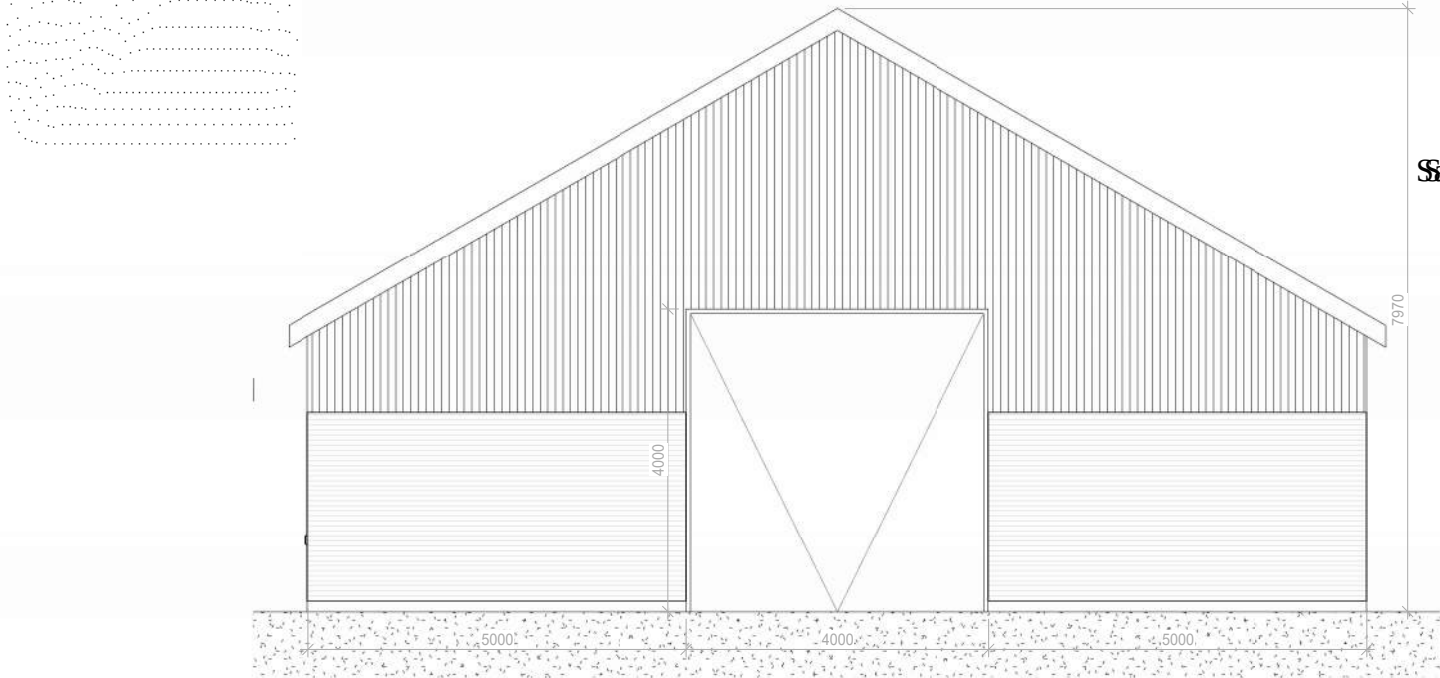
Myndighed - Facade mod vest - Fremtidig | 1 : 100
