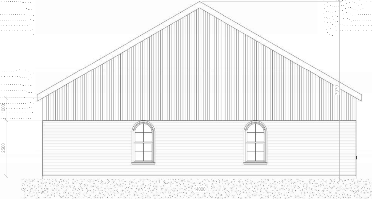
Myndighed - Facade mod øst - Fremtidig | 1 : 100
