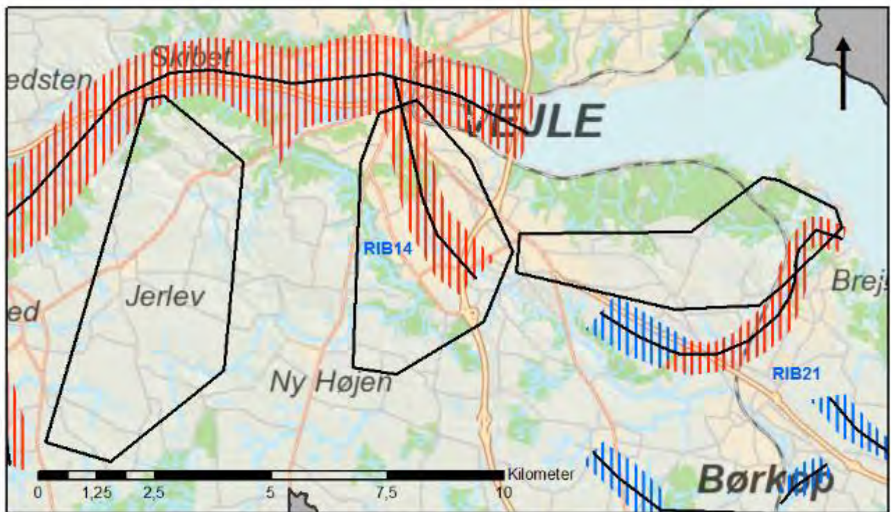
Kort over RIB14 (veldokumenteret delvist begravet dal) og RIB21 (deltvist begravet dal) som længst mod vest er svagt dokumenteret og mod øst veldokumenteret (GEUS 2009)
