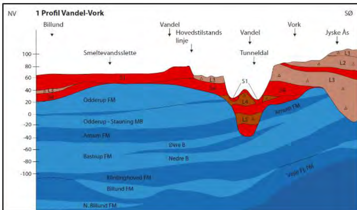
Geologisk profil (forsimpler) fra NV til SØ med tunneldal, begravet dal, bakkeø ved Vandel, smeltevandsslette mellem Vandel og Billund og del af Jyske Ås ved området omkring Vork
