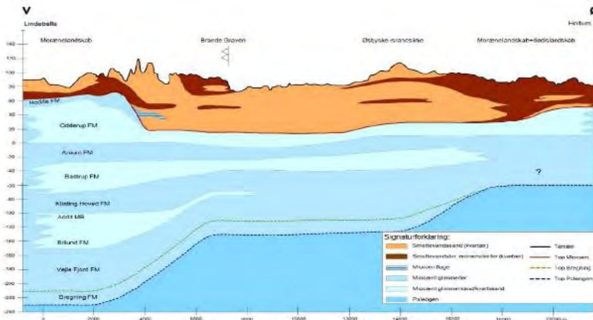
Geologisk profil (forsimpler), der viser Hvejsel-området overordnede geologiske opbygning fra V til Ø med Brande Graven, randmorænestrøget i den østlige del af Gårup-området og den vestlige del af Bredsten-området (Østtyske israndslinie) og dødislandskabet i Hvejsel
