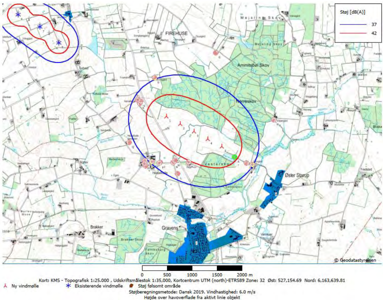
Figur 7.1.3: Støj beregning for udendørs støj ved 6 m/s fra nye og blivende vindmøller. 42 dB(A) er støjkravet for enkeltliggende nabobeboelser, markeret med rødlig cirkel og et bogstav, der henfører til en adresse med oplysninger i støj beregningsrapporterne, der vedlagt som bilag. 37 dB(A) støjkravet for støjfølsomme områder. De støjfølsomme områder er vist med rødbrun farve.
