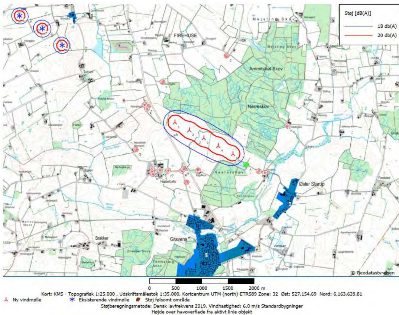
Figur 7.1.5: Støjregning for lavfrekvent støj ved 6 m/s fra nye og blivende vindmøller. 20 dB(A) er støjkravet for enkeltliggende nabobeboelser, markeret med rødlig cirkel og et bogstav, der henfører til en adresse med oplysninger i støjregningsrapporterne, der vedlagt som bilag. 20 dB(A) er støjkravet for støjfølsomme områder.
