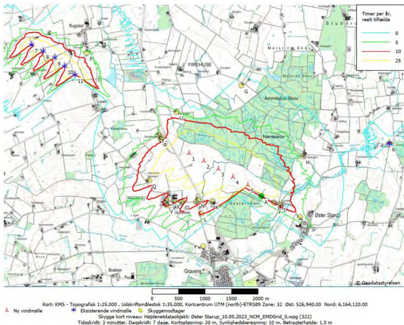
Figur 7.2.2: Kort over udbredelse af beregnet skyggekast fra vindmøller, uden etablering af skyggestop på vindmøllerne. Linjerne viser skyggekast i timer pr. år beregnet som reel værdi, Rød linje angiver den anbefalede grænseværdi på 10 timer pr. år. Nabobeboelser er markeret med en gulgrøn cirkel og et bogstav, der henfører til en adresse med oplysninger i skyggeberegningerne, der er vedlagt som Bilag 3.
