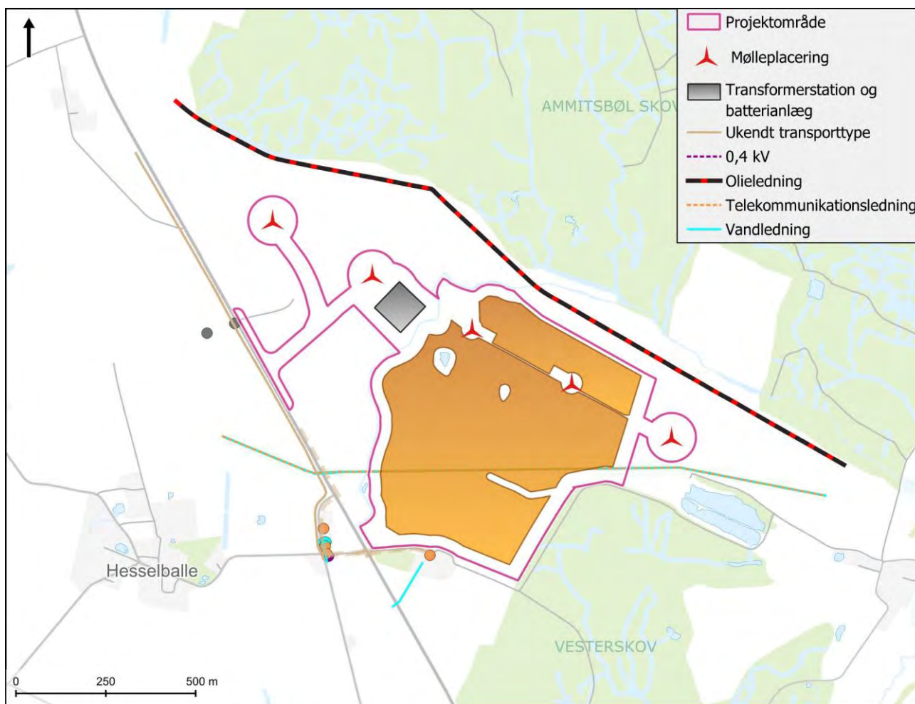
Figur 5.8.1 Tekniske anlæg (LER oplysninger) i projektområdet.
