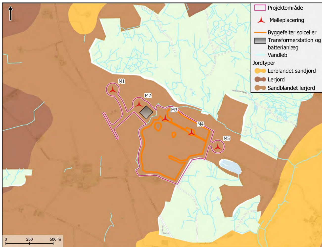
Figur 7.6.4 Jordtypekort.
