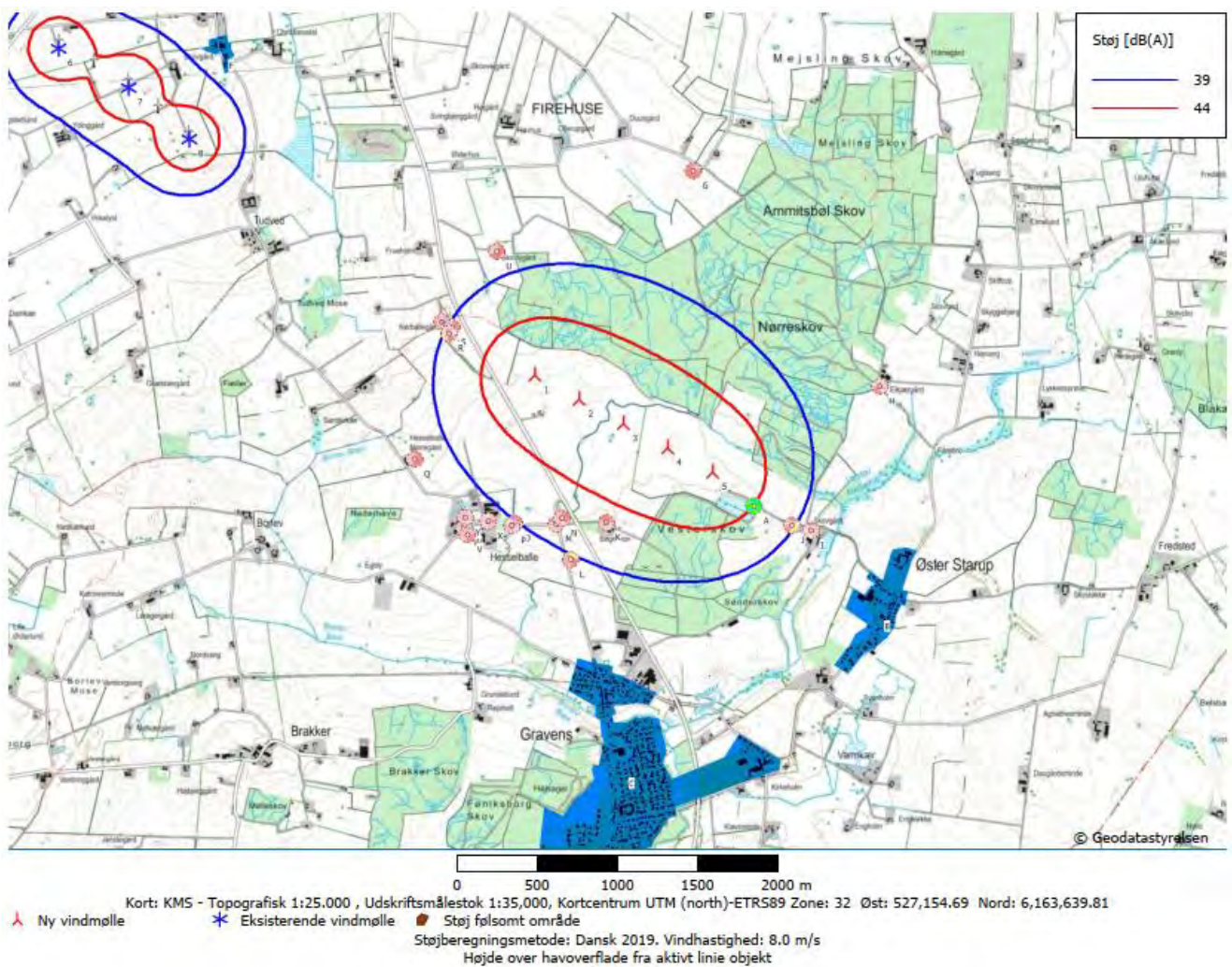
Figur 7.1.4: Støjberegning for udendørs støj ved 8 m/s fra nye og blivende vindmøller. 44 dB(A) er støjkravet for enkeltliggende nabobeboelser, markeret med rødlig cirkel og et bogstav, der henfører til en adresse med oplysninger i støjberegningsrapporterne, der vedlagt som bilag. 39 dB(A) er støjkravet for støjfølsomme områder.
