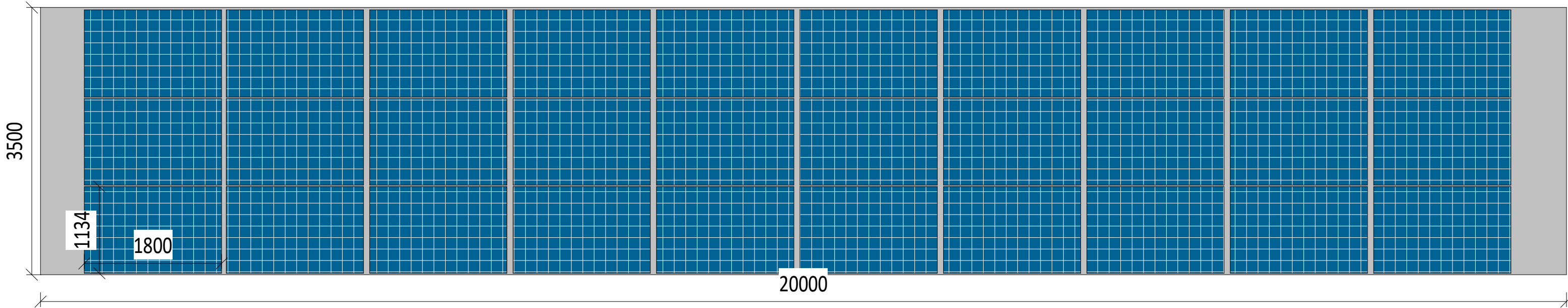
Plan 1:50
