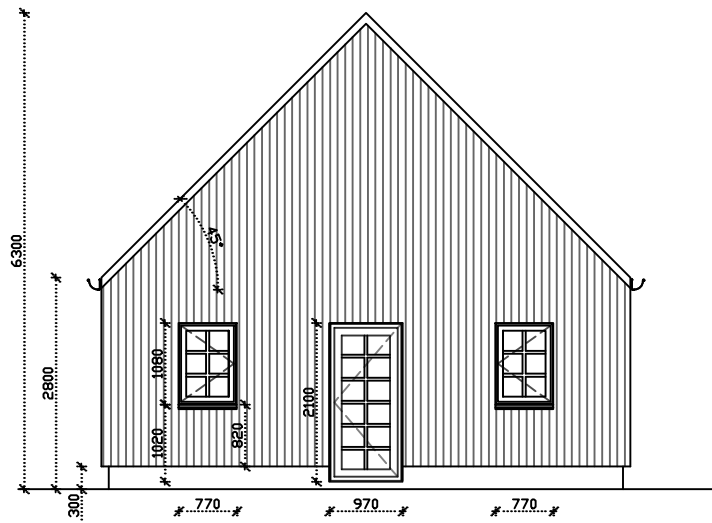
FACADE NORD
