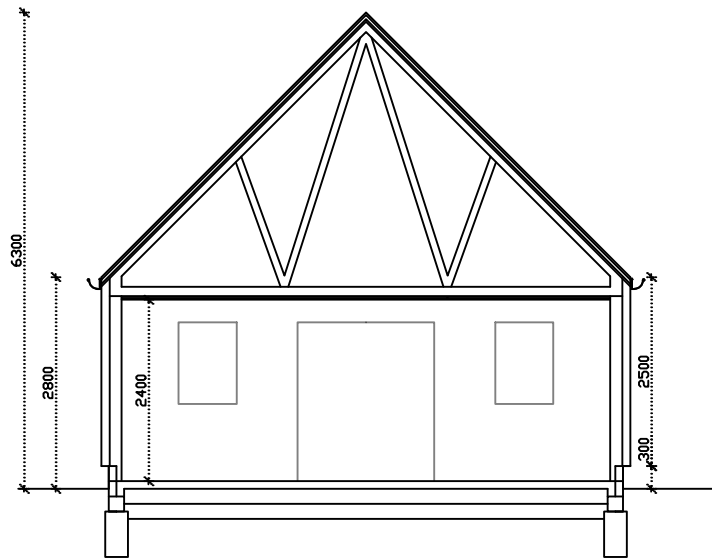
PRINCIPSNIT
