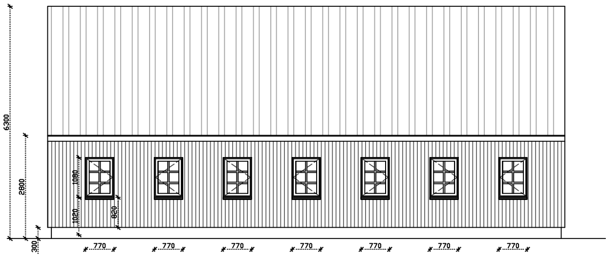
FACADE ØST
