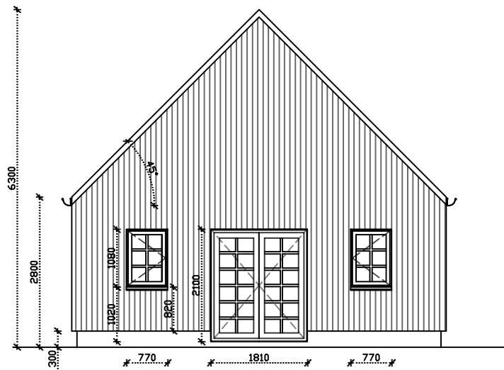
FACADE SYD
