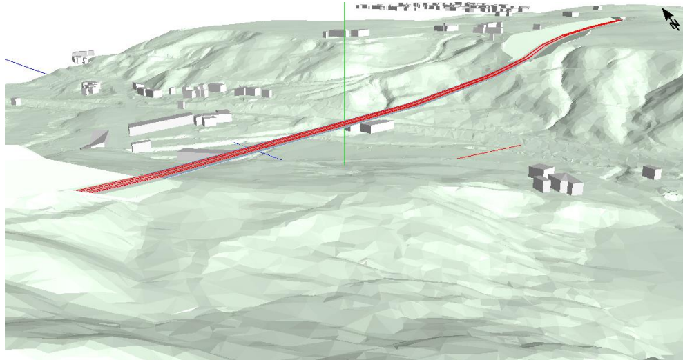
Figur 5 Udsnit af støjmodellens topografi i 3D, krydsning af Grejsdalen linje 1 (lav bro).
