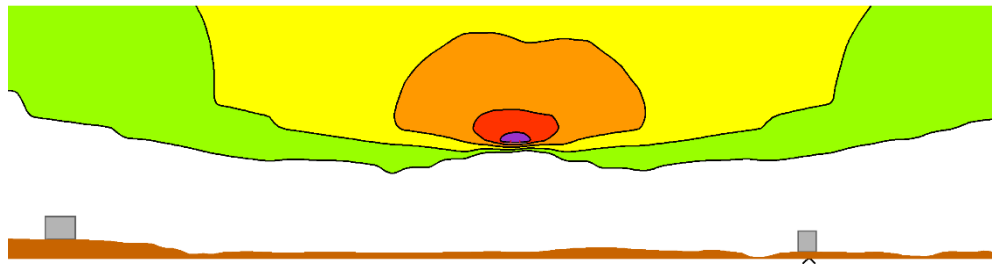
Figur 7 Vertikal støjudbredelse i udvalgt tværsnit, krydsning af Grejsdalen linje 1 (lav bro).
