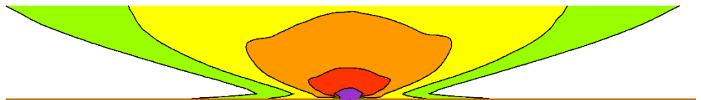
Figur 22 Vertikal støjudbredelse i udvalgt tværsnit, vej i 2 m afgravning og med 1 m høj jordvold.
