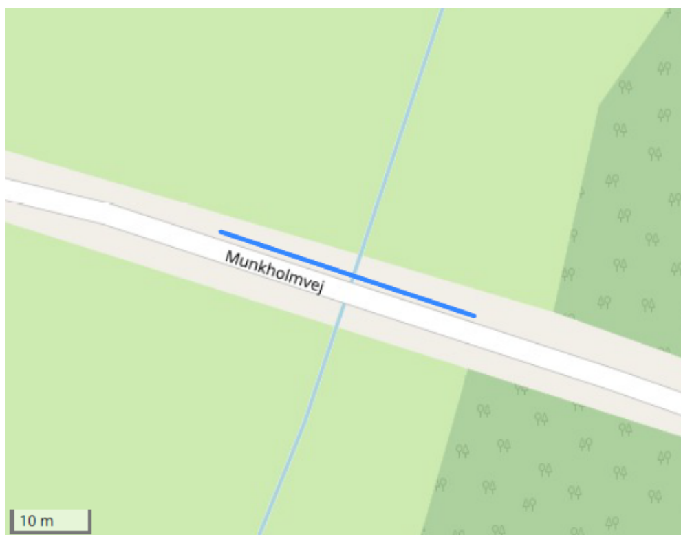
Figur 2: Kortudsnit af underboringens placering ved krydsningen af Farre Bæk.
