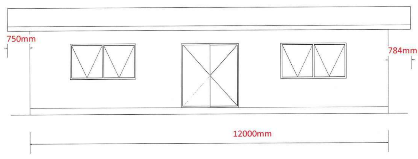
Nord facade
