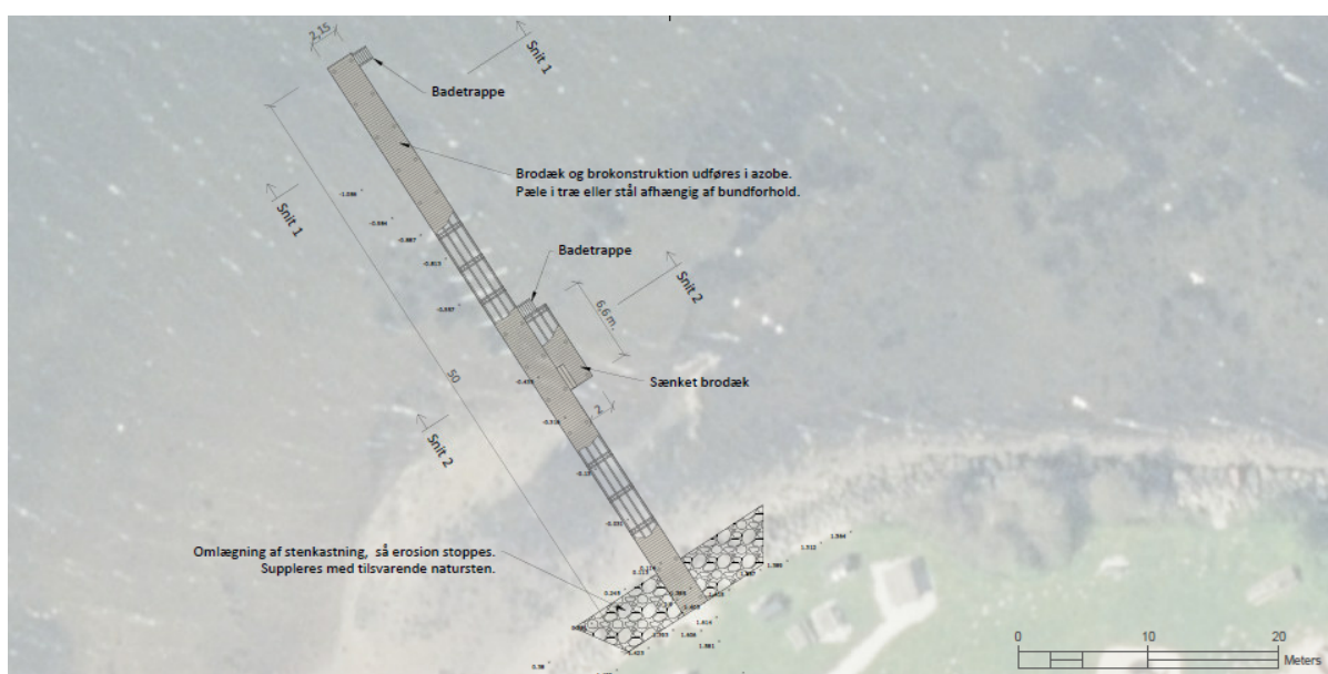
Figur 2. Planskitse for broen.
