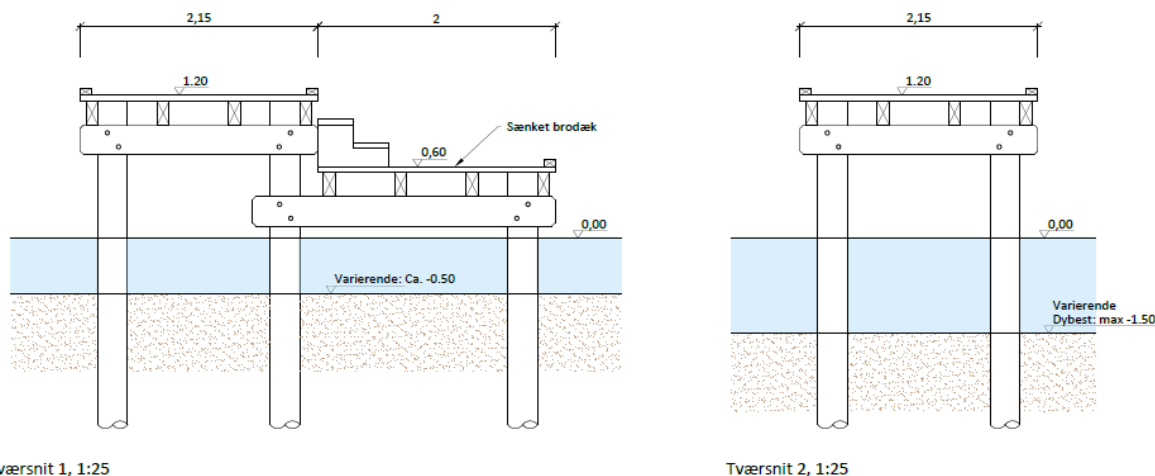
Figur 3. Tværsnit af broen.
