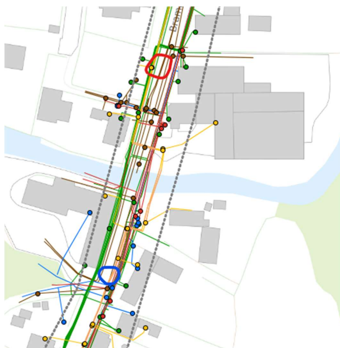
Figur 2: Kortbilag - Oversigtskort af projektområde. Start hul markeret med blå cirkel og modtagerhul markeret med rød cirkel.
