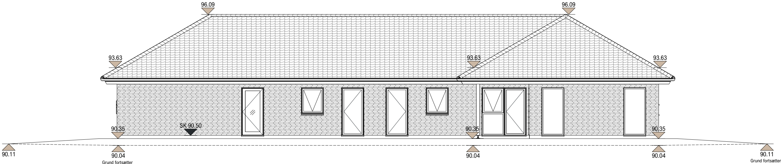
Facadeopstalt 2 (Syd)
