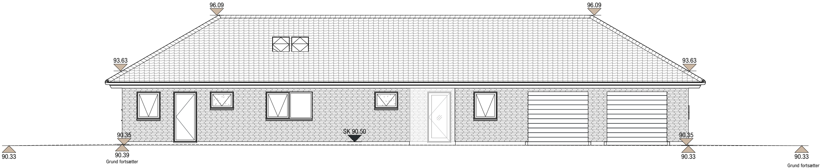
Facadeopstalt 4 (Nord)
