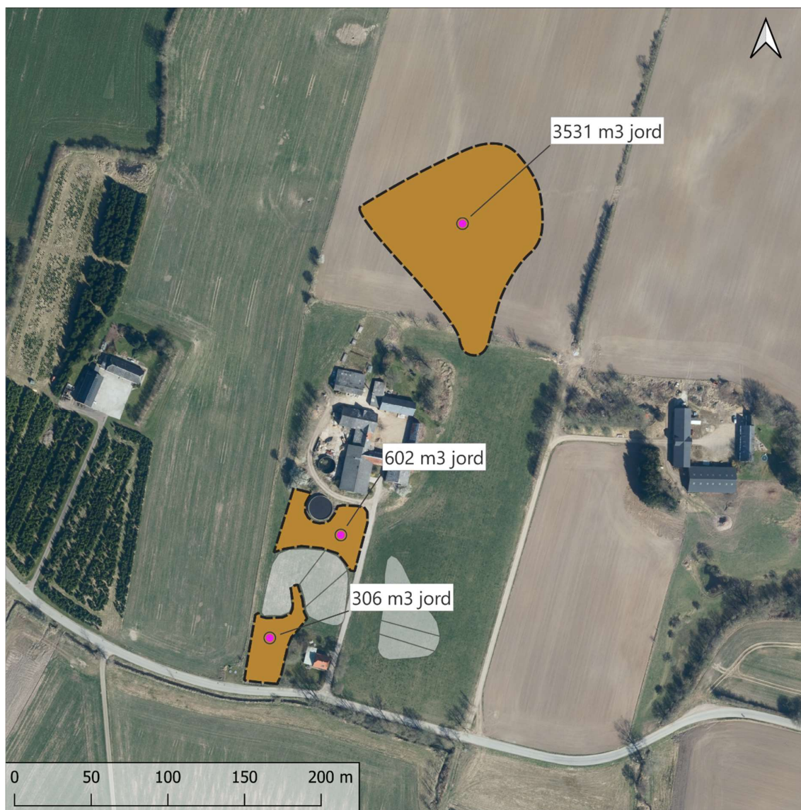
Figur 6: skitse over minivådområde og områder for placering af overskudsjord.
