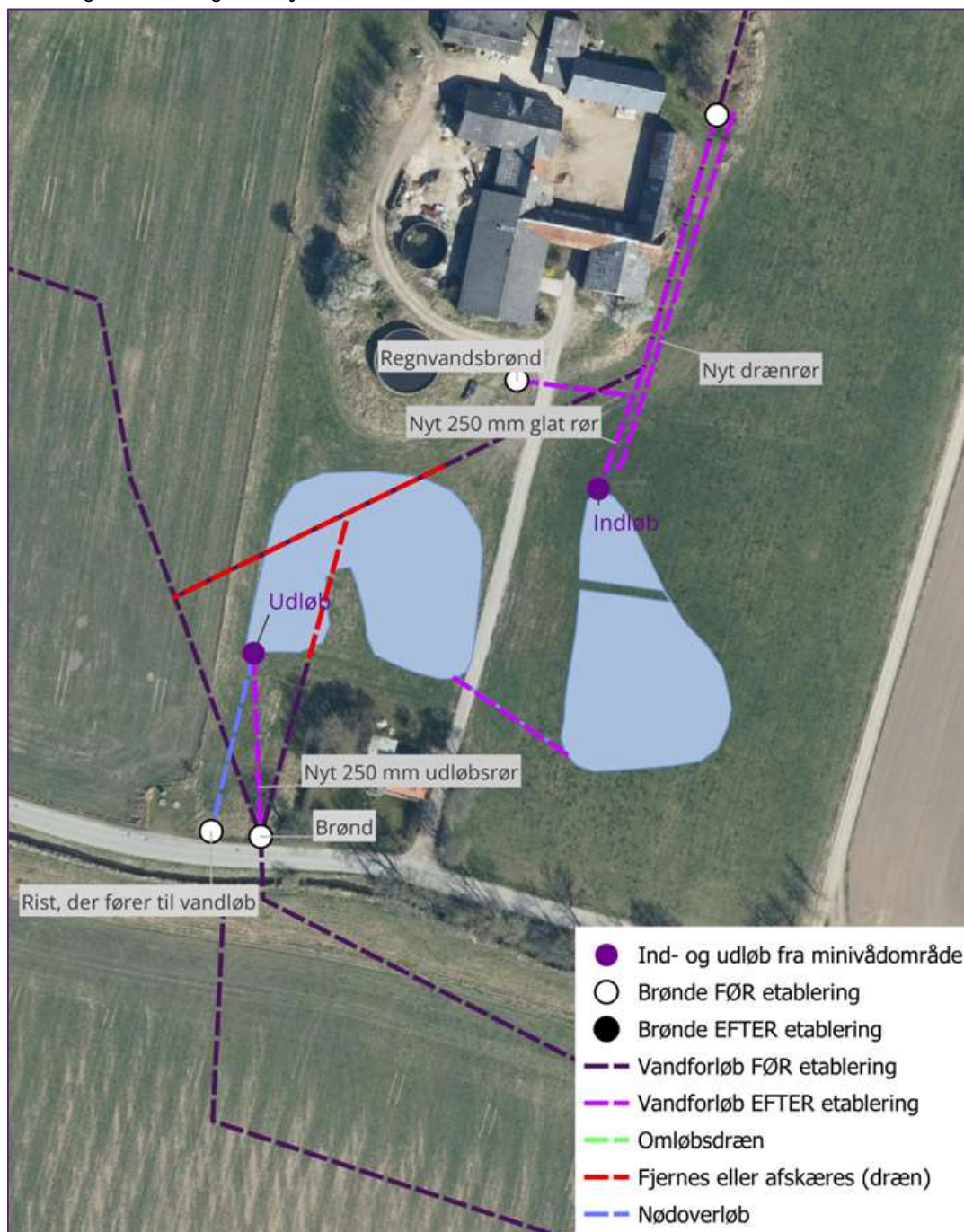
Figur 4.: Drænforløb før og efter etablering.
