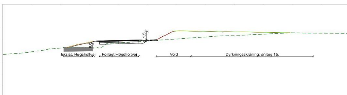
Illustration 2. Snit gennem volden ved den blå linje på illustration 1.
