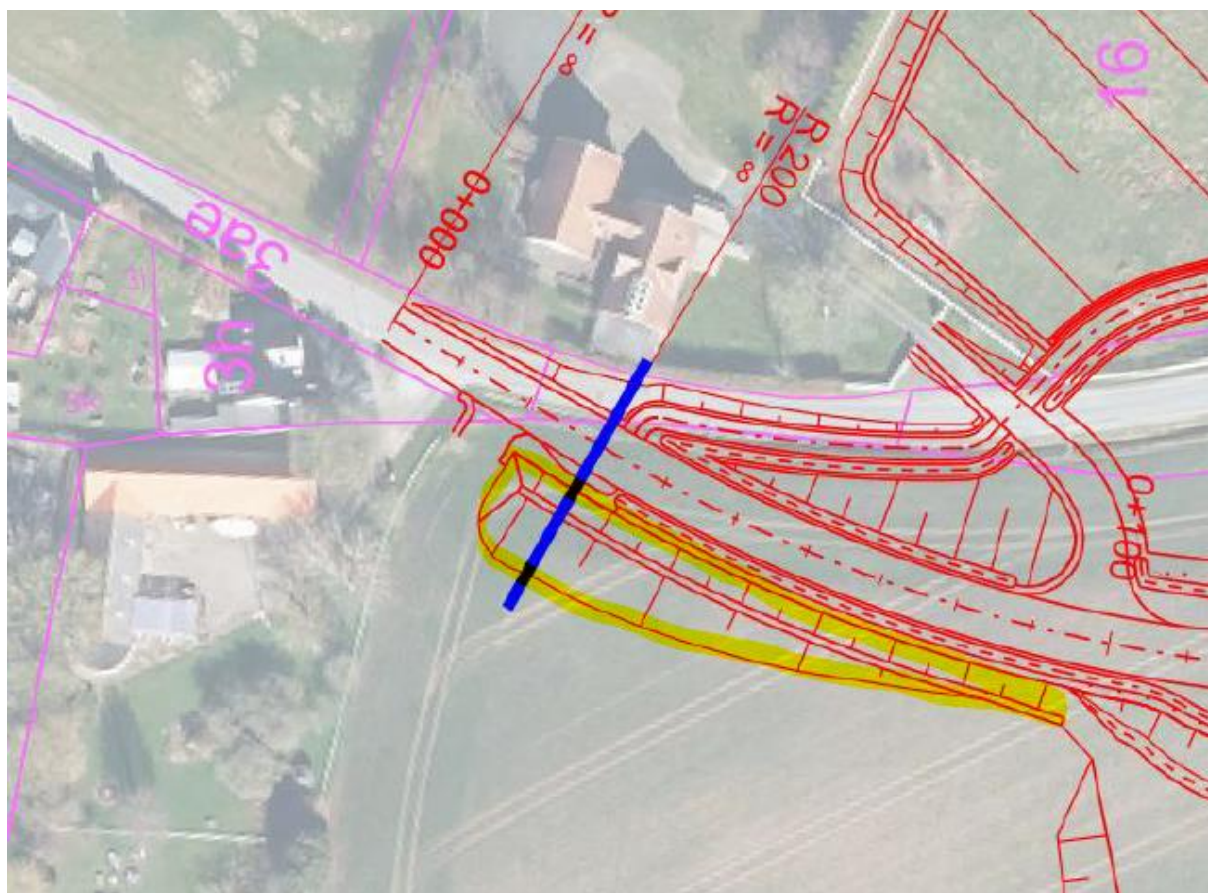
Illustration 1. Jordvolden er markeret med gul. Snit gennem volden ses som den blå linje.
