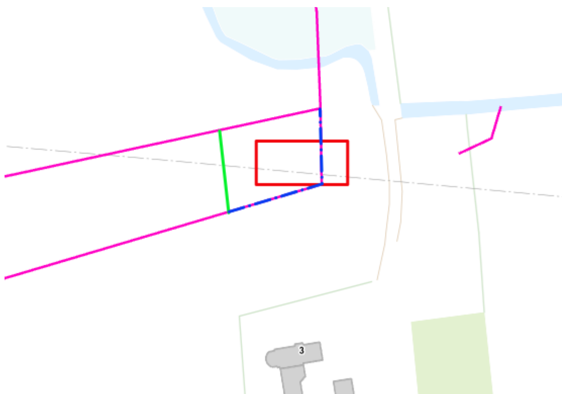
Figur 2: Omlægning af dræn. Det eksisterende hoveddræn ansøger ønsker fjernet er markeret med stiptet blå, og det nye drænforløb er markeret med grøn.
