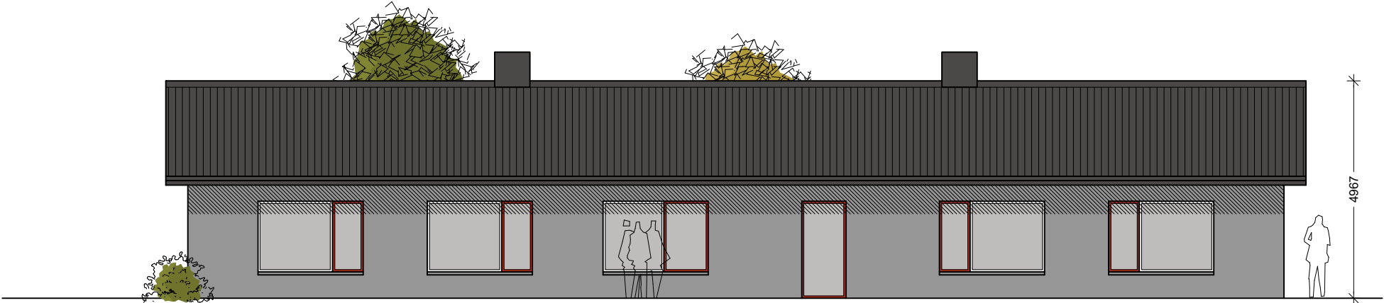
Facade mod syd
