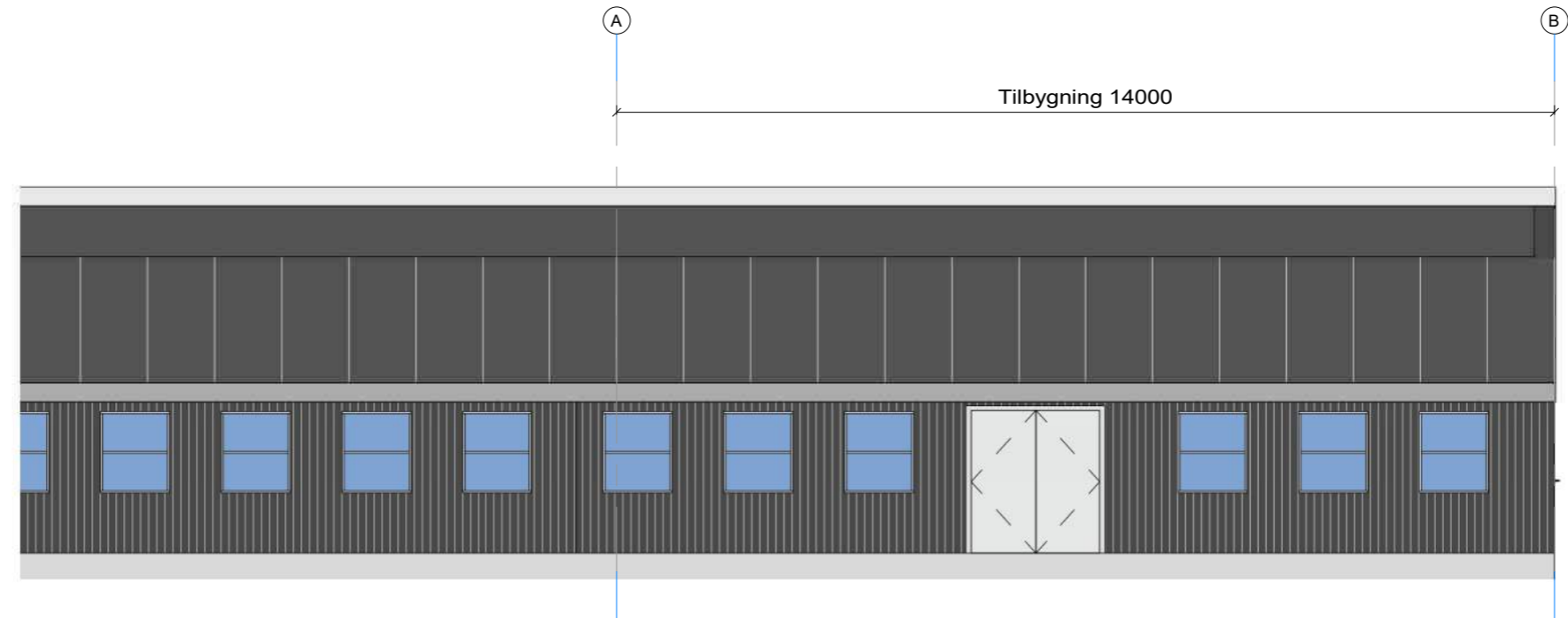
Facade mod øst 1 : 100
