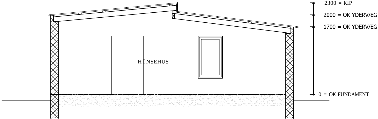
SNIT A-A
