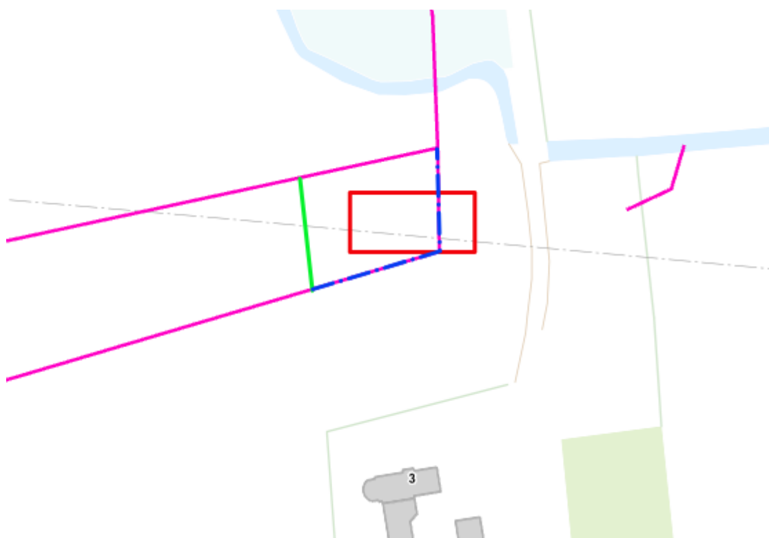
Figur 2: Omlægning af dræn. Det eksisterende hoveddræn ansøger ønsker fjernet er markeret med stiplede blå, og det nye drænforløb er markeret med grøn.
