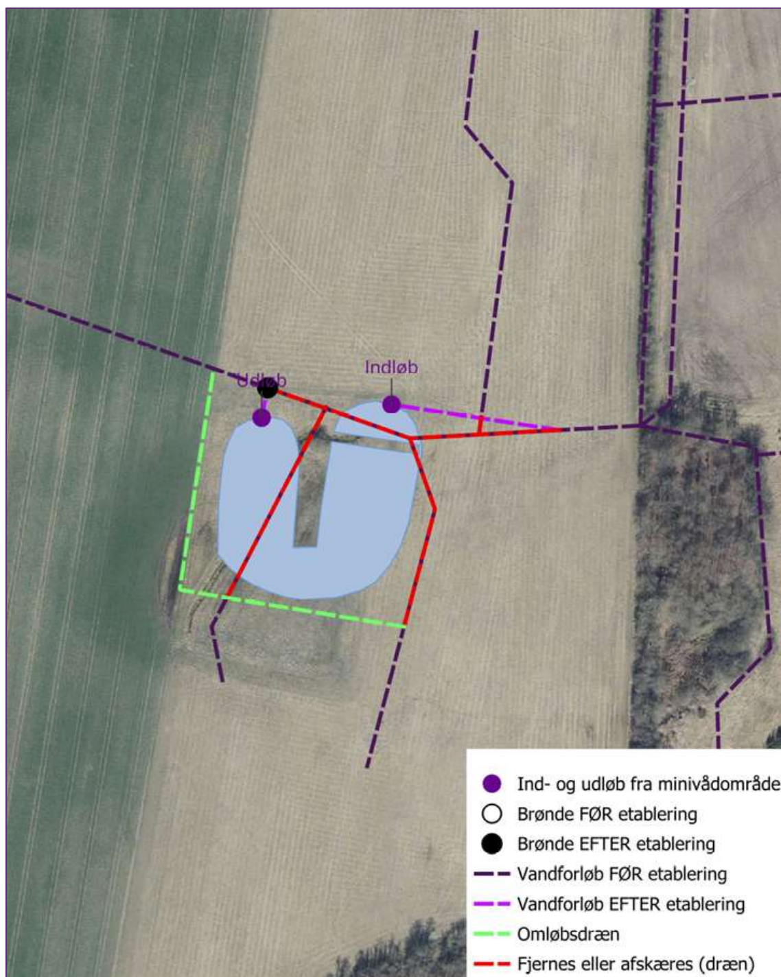
Figur 6.: Drænforløb efter etablering.
